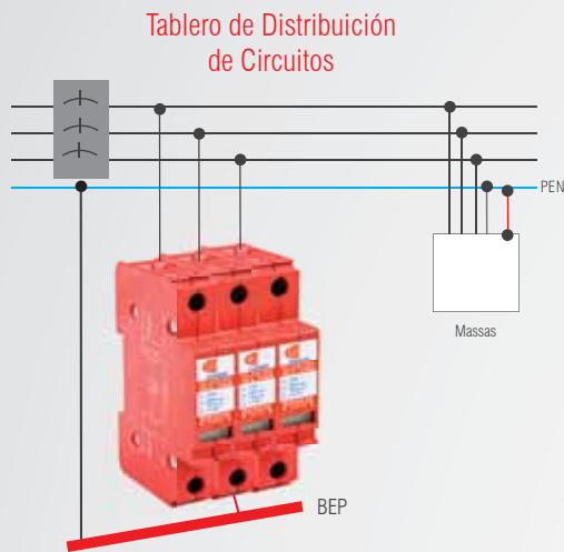
Ejemplo de aplicación de DPS en el esquema tipo TN-C.
