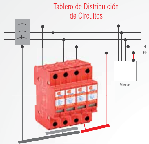
Ejemplo de aplicación de DPS en el esquema de tierra tipo TN-S, en tablero secundario.
