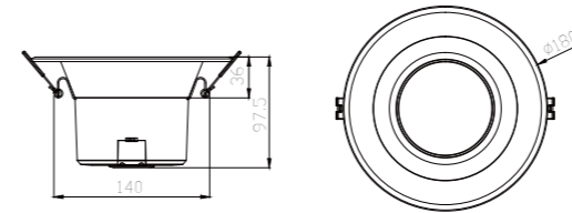
Size:(mm) 15W / 18W
