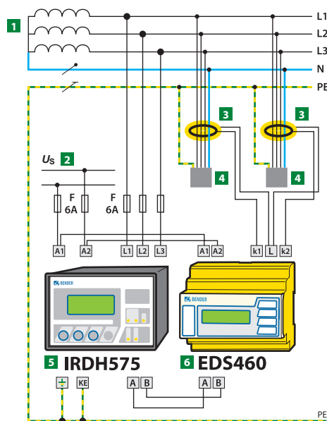
Sistema EDS con IRDH575, EDS460 y transformadores toroidales W... en el sistema 3AC
