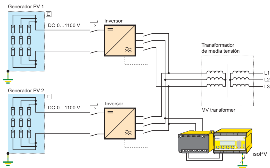
Varios generadores de PV aislados de tierra (sistema IT) con tensión nominal \leq DC 1100 V como sistema acoplado e ISOMETER® isoPV con acoplador AGH-PV
