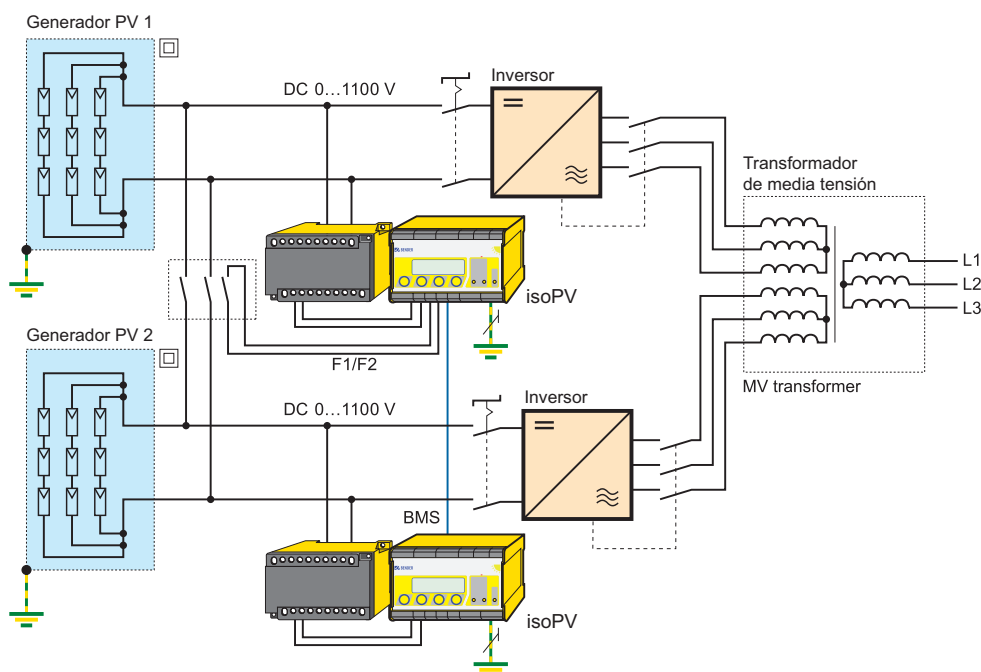
Generador de PV aislado de tierra (sistema IT) con tensión nominal \leq DC 1100 V e ISOMETER® isoPV con acoplador AGH-PV
