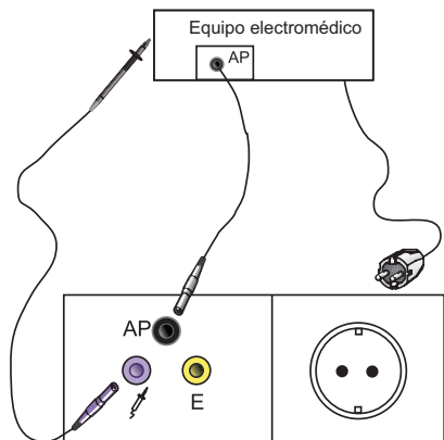
Conexión de equipos electromédicos con conexión por enchufe
