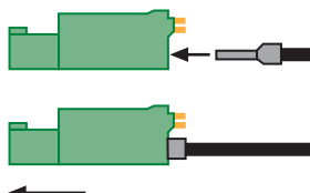
Conectar los conductores
