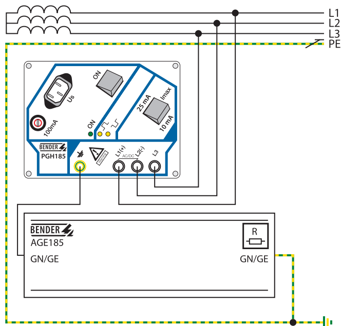
Aparato de prueba de fallos de aislamiento PGH185 y acoplador AGE185
