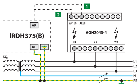
ISOMETER® IRDH375 con acoplador AGH204S-4
